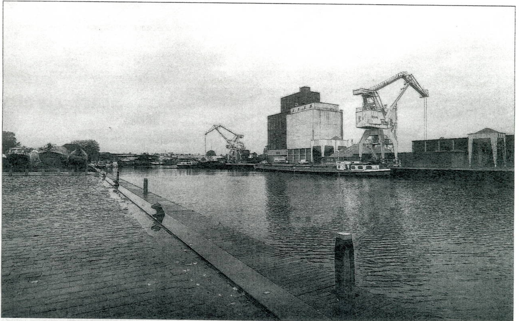
Uitbaggeren van het kanaal is bittere noodzaak om de haven van Enschede bereikbaar te houden. Ook de kades kampen met achterstallig onderhoud. Een deel van de kades, zoals op deze foto de Handelskade, is inmiddels vernieuwd. foto Tim Uunk
